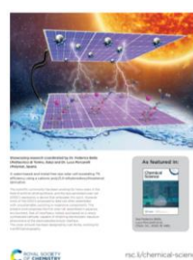
Chem. Sci. 11 (2020) 1485-1493
